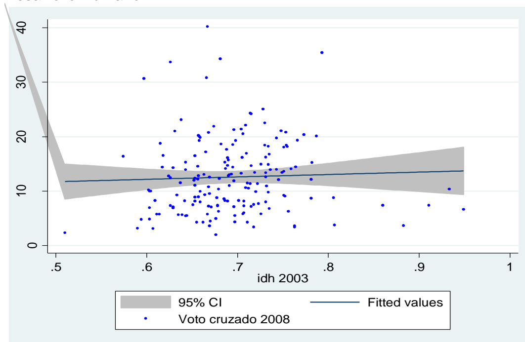
Gráfico 5. Diagrama de dispersión entre voto cruzado 2008 e Índice de Desarrollo Humano
