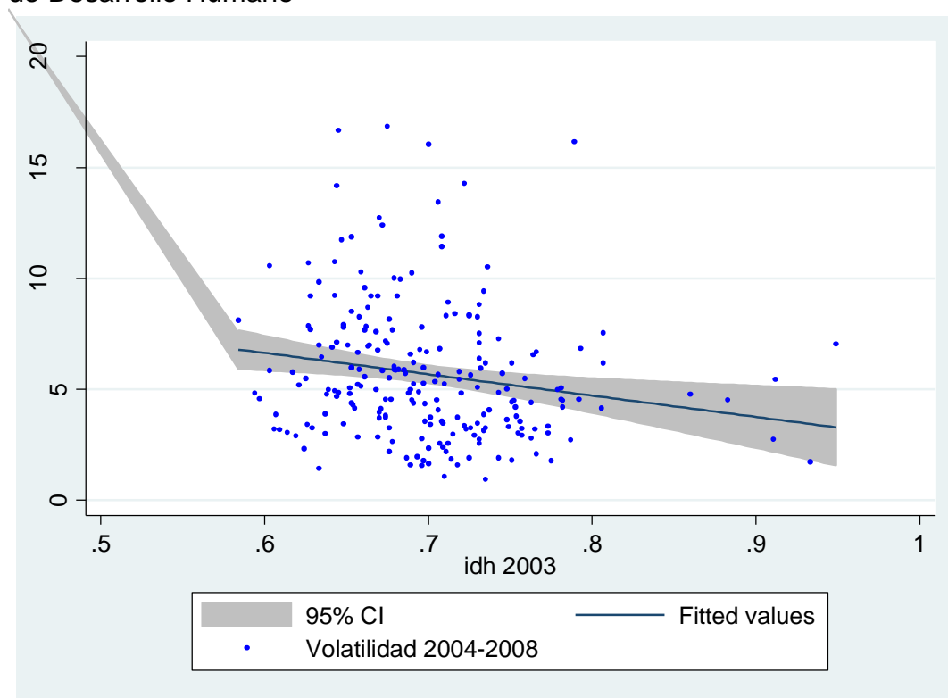
Gráfico 4. Diagrama de dispersión entre volatilidad electoral 2008-2004 e Índice de Desarrollo Humano
